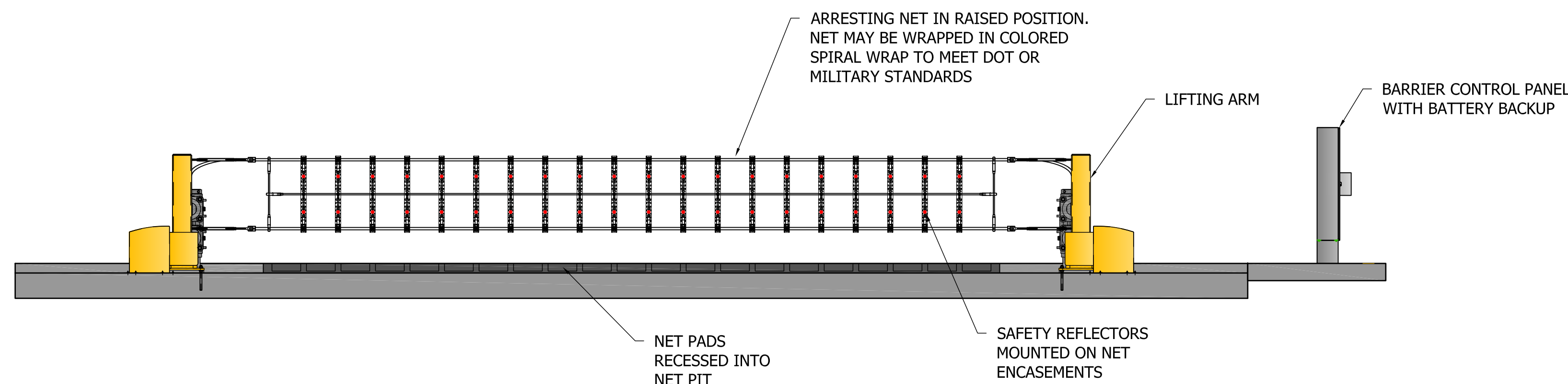
A-1 - ELEVATION VIEW SCALE: 1/4" = 1'-0"
